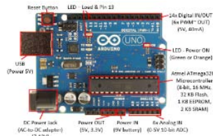
Gambar 6. Arduino Uno
