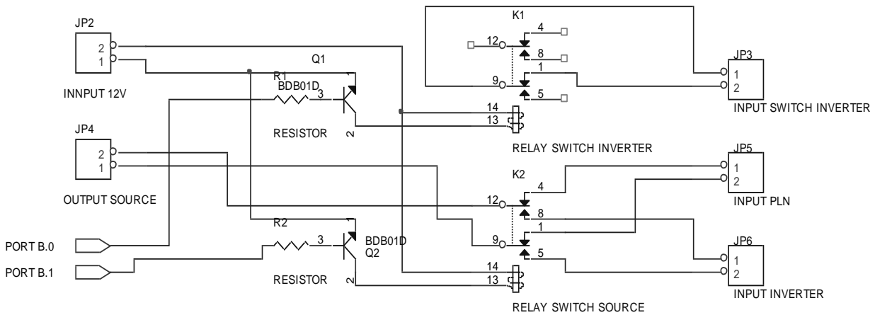
Gambar 9. Rangkaian Relay
