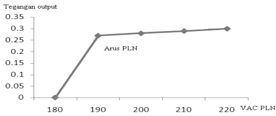
Gambar 21. Grafik Pengukuran Arus PLN
