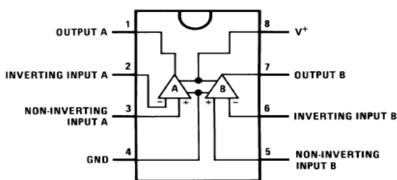
Gambar 2. IC LM358
