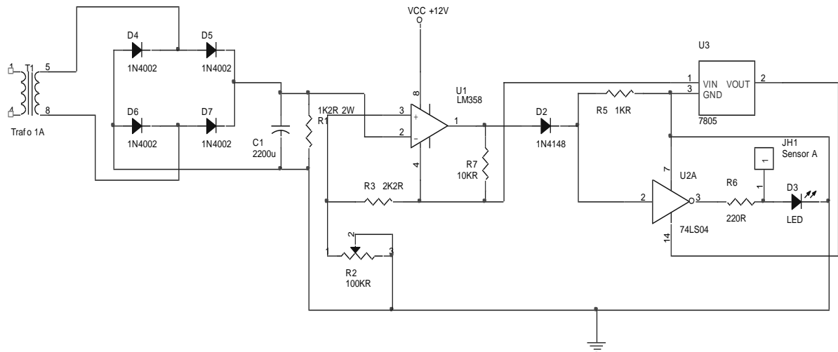
Gambar 8. Rangkaian Sensor Tegangan
