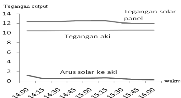
Gambar 20. Grafik Pengukuran Pengisian Aki
